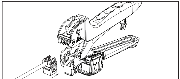
Step 3. Insert the HD module.
