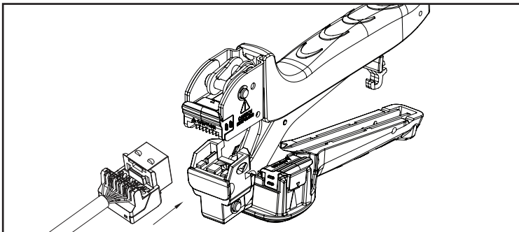
Step 2. Insert the EZ module.
